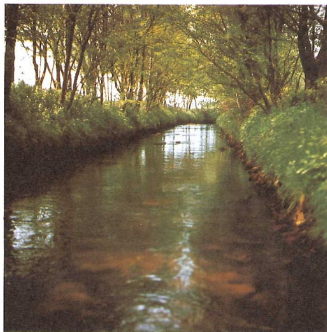
Ausbaustrecke mit planmäßig angelegtem Ufergehölzbestand. Vorherrschende Baumart ist die Schwarzerle. Im beschatteten Gewässerbett entwickelt sich kein störender Aufwuchs, so daß sich hier Unterhaltungsarbeiten erübrigen.
