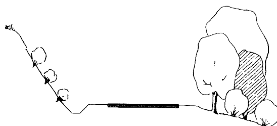
⑥ Sicherung der Anschnittsböschung durch Buschlagen, Bepflanzung der Auftragsböschung
