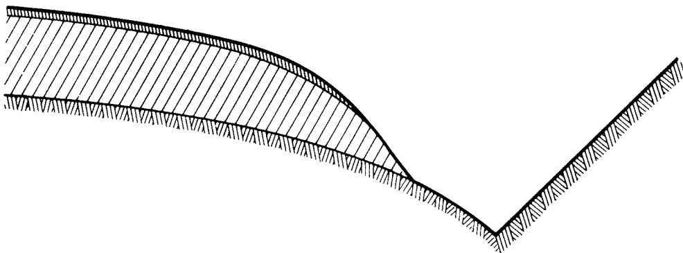
e) Rinnenbordstein
