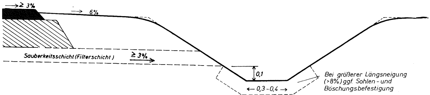
a) Seitengraben
