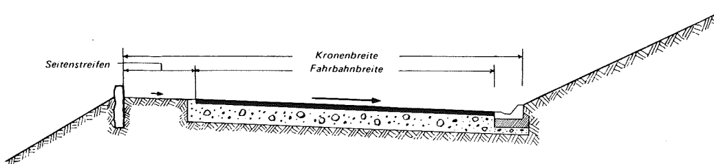
d) Wirtschaftsweg mit bergseitig geneigter befestigter Fahrbahn und Rinne
