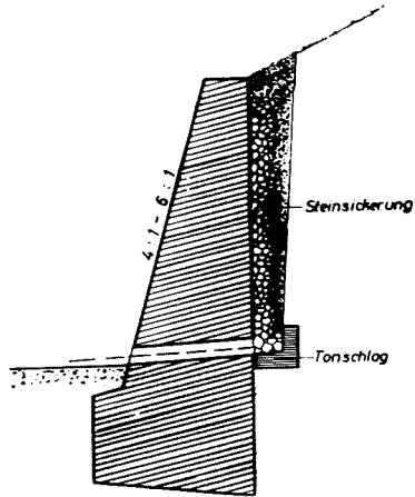
Schwergewichtsmauer
