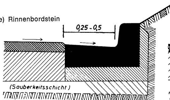
f) Schrägbord mit Längssickerung
