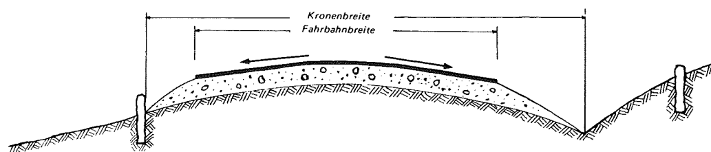
f) Fahrbahn mit gewölbter Fahrbahn und Spitzgraben
