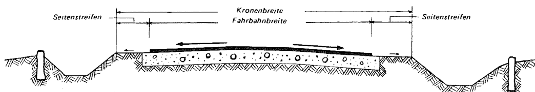
e) Wirtschaftsweg mit zweiseitig geneigter Fahrbahn und Seitengraben
