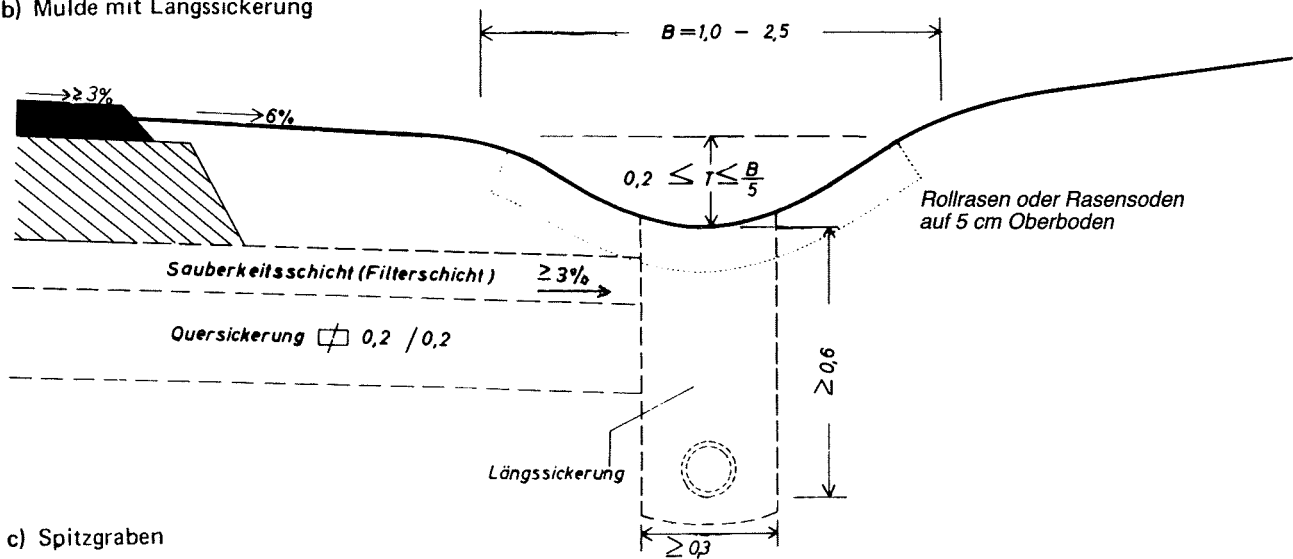
b) Mulde mit Längssickerung
