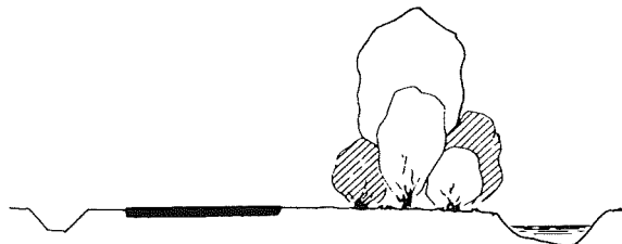
② Durch Anlehnen der neuen Wegtrasse an den Bachlauf entstehen bei gleichzeitig besserer Wegführung zusammenhängende Grundstücke. Die Restflächen zwischen Weg und Bach werden bepflanzt. Einer Regulierung dieses Baches bedarf es nicht.
