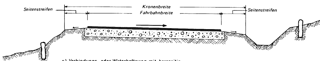
c) Verbindungs- oder Wirtschaftsweg mit bergseitig geneigter befestigter Fahrbahn und Seitengraben
