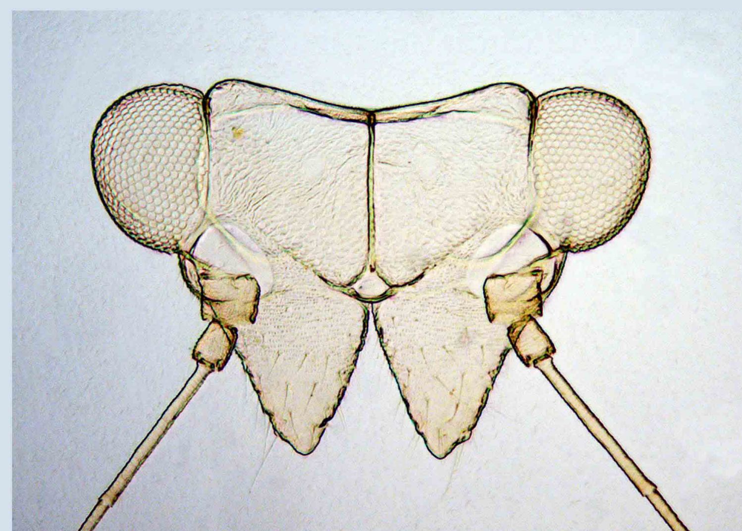
Kopf
