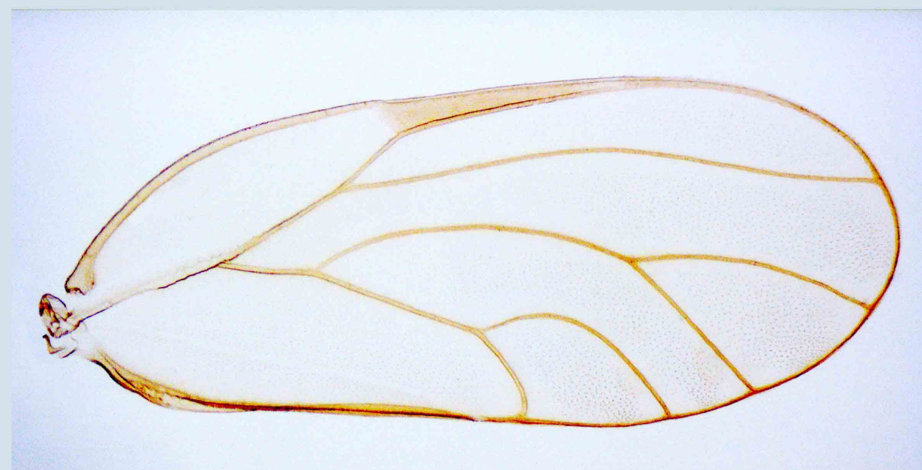
Vorderflügel
